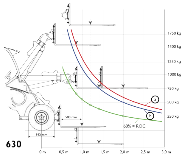
Wykres obciążenia 630/635/640
